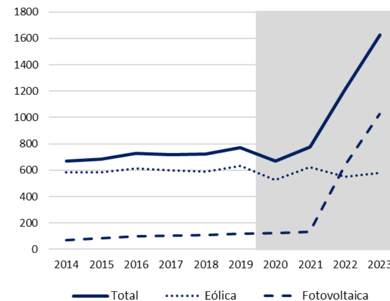
Produção de energia elétrica a partir de fontes renováveis (Gwh)
